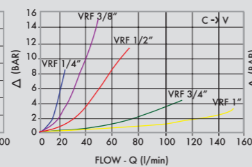
STROZZATORE TUTTO APERTO - FULLY OPENED THROTTLE
